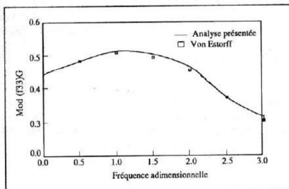
Figure 4 : Comparaison avec des résultats publiés. Conditions aux limites relâchées (fondation superficielle).
