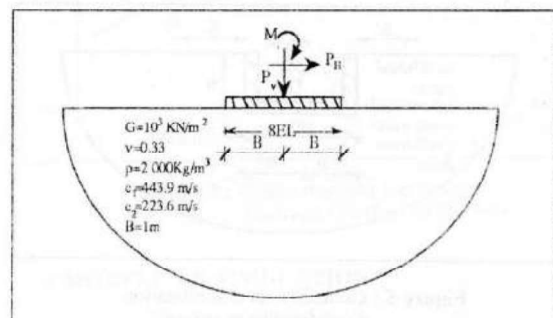
Figure 3 : Discrétisation et géométrie d'une fondation superficielle.
