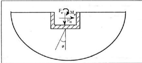
Figure 1 : Géométrie et notation d'une fondation enterrée.
