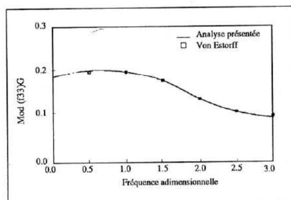
Figure 6 : Comparaison avec des résultats publiés. Conditions aux limites parfaites (fondation enterrée E/B = 1 ).
