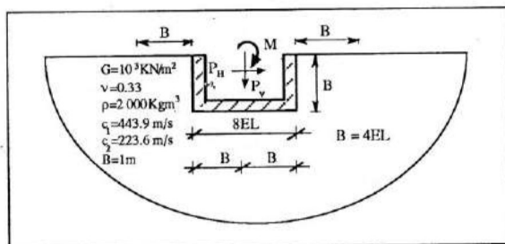
Figure 5 : Géométrie et discrétisation d'une fondation enterrée.
